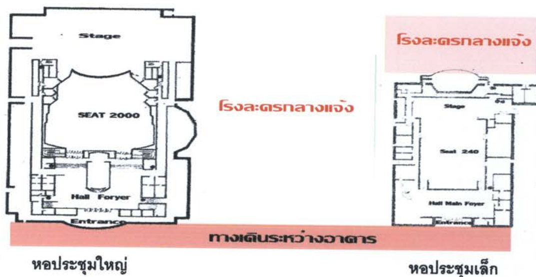
ภาพที่ 2.30 แสดง Lay Out Of Plan
