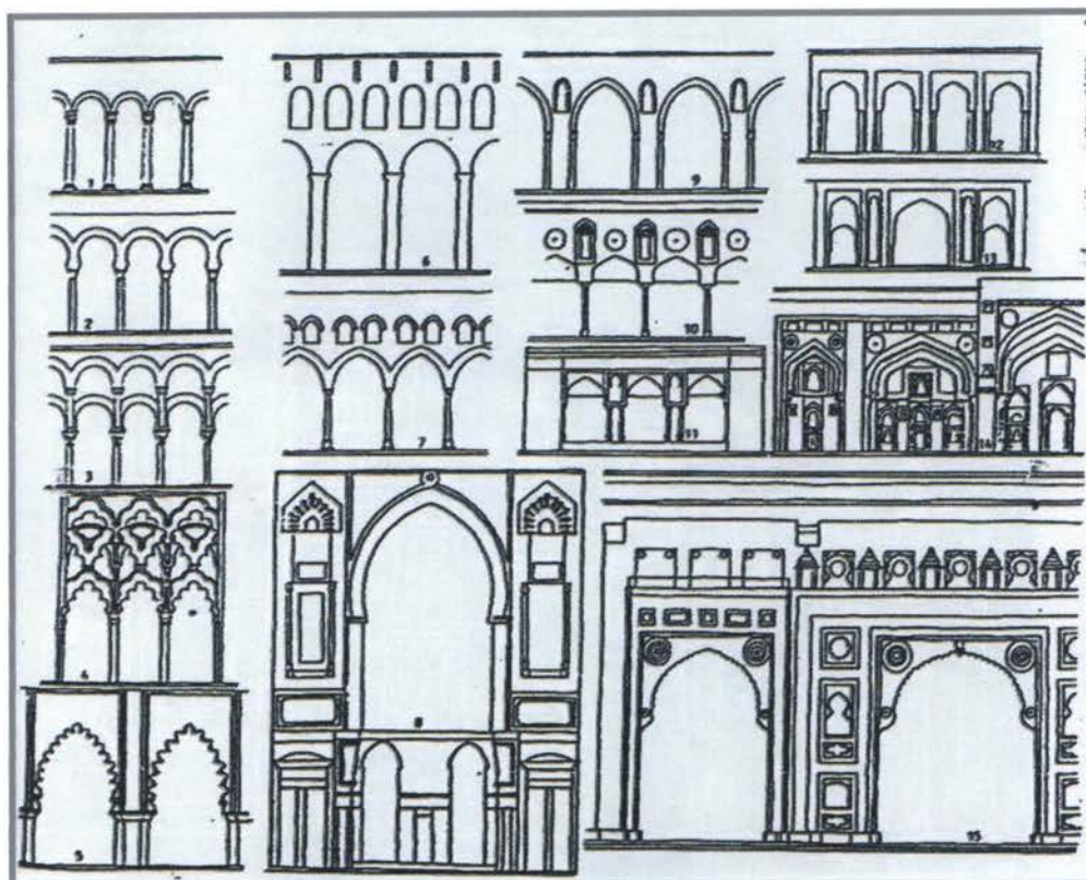
ภาพที่ 2.18 แสดงลักษณะของรูปแบบ Arch ของสถาปัตยกรรมอิสลาม
