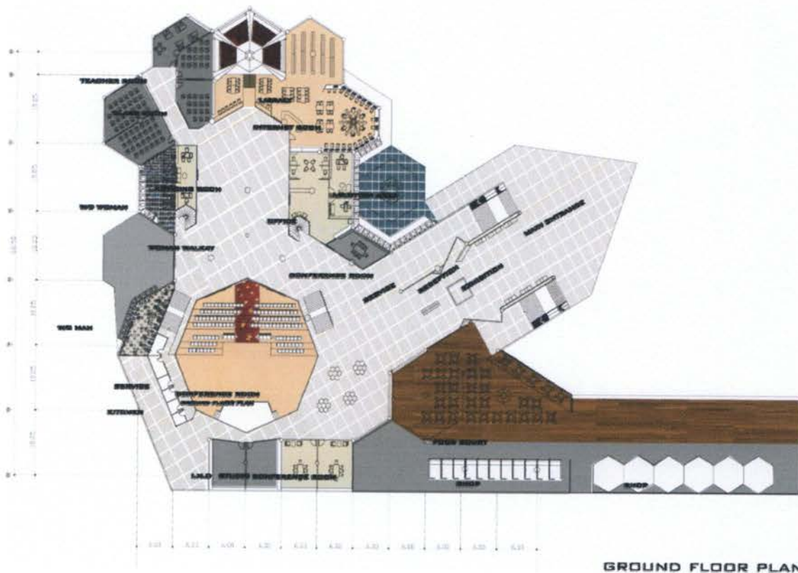
ภาพที่ 5.2 ผังพื้น แสดงทางเลือกที่ 2 ที่มา : จากการศึกษาและวิเคราะห์
