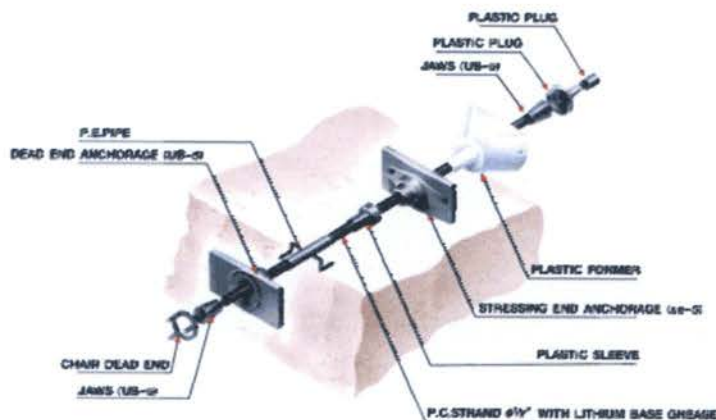
ภาพที่ 3.17 แสดงลักษณะการรับแรงดึงของพื้น Post tensioned
