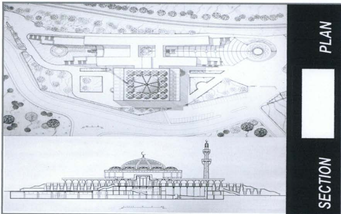
ภาพที่ 2.49 แปลนอาคาร ISLAMIC CULTURAL CENTRE OF ROME ที่มา : วิทยานิพนธ์มูลนิธิเพื่อศูนย์กลางอิสลามแห่งประเทศไทย ห้องสมุด สถาปัต
