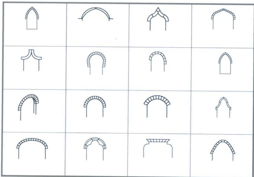
ภาพที่ 2.15 แสดงลักษณะของรูปแบบ Arch ของสถาปัตยกรรมอิสลาม
