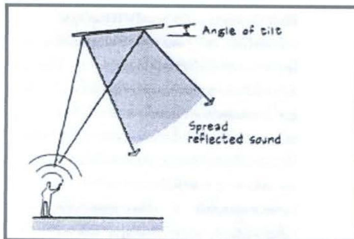
ภาพที่ 3.19 แสดงConcave Reflector
